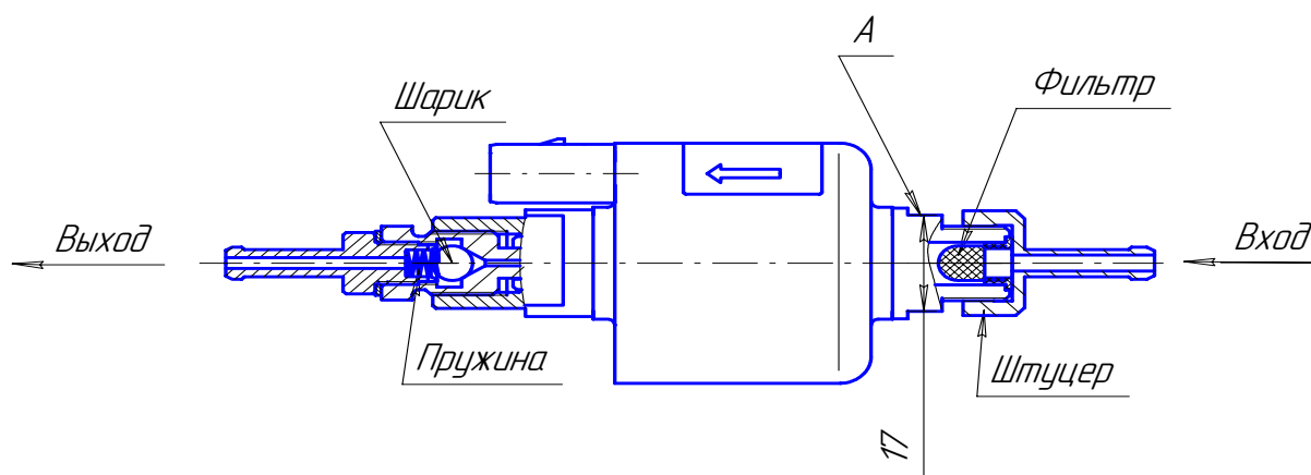
Рис. 9.1 – Топливный насос
