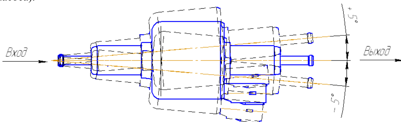
Рис. 7.7 Допустимое монтажное положение бензинового топливного насоса (производства Thomas Magnete)
